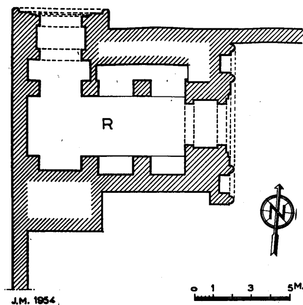
Fig. 3. — Entrée de la première enceinte, plan.
