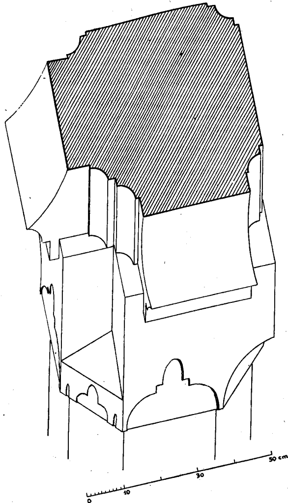
Fig. 11. — Pavillon, chapiteau et départs d'arcs du patio.
