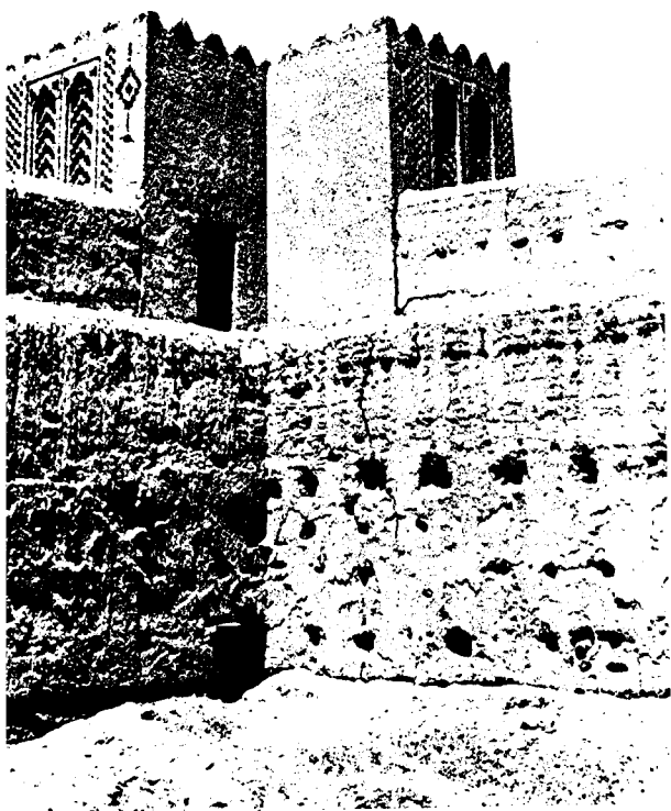
15 - Abbar ; tour NW de la qasba, vue de l'intérieur.
