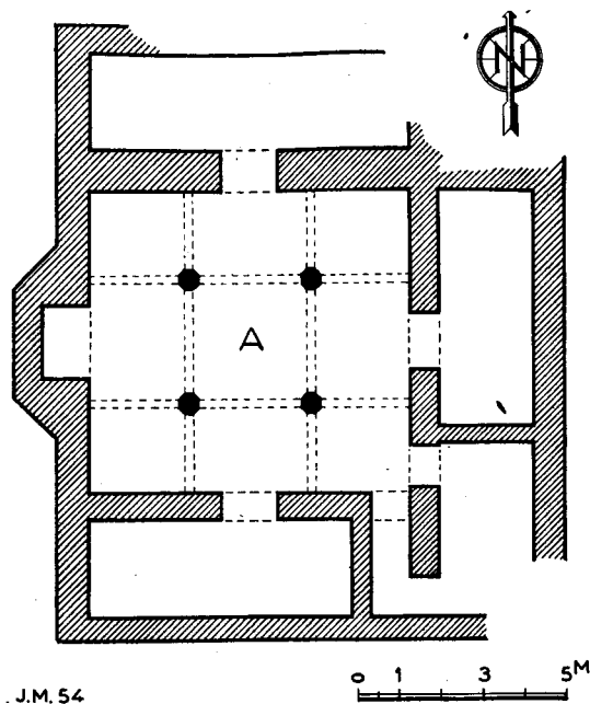
Fig. 9. — Pavillon, plan.
