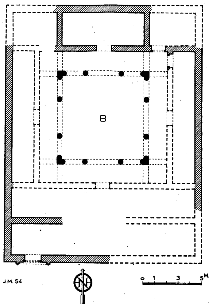
Fig. 7. — Petit Palais, plan.
